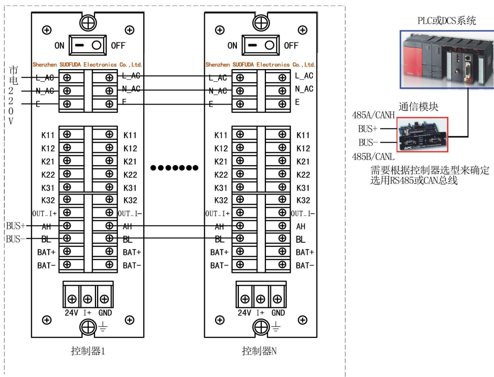
（图 16、报警控制器输出的总线信号与消防控制主机、DCS 或 PLC 的连接方法）
