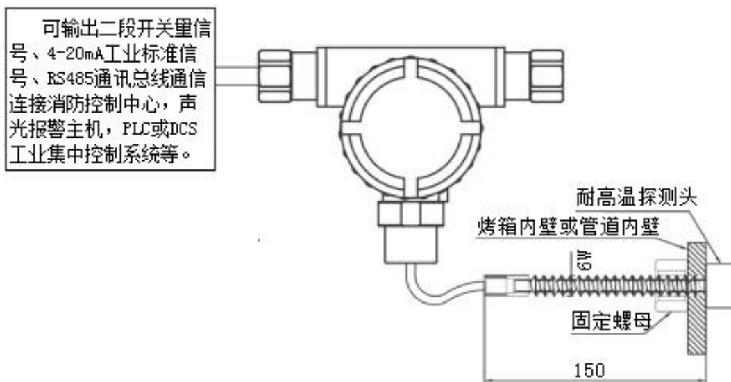
（图 5、使用于高温、管道等特殊场合的气体探测器安装图）
