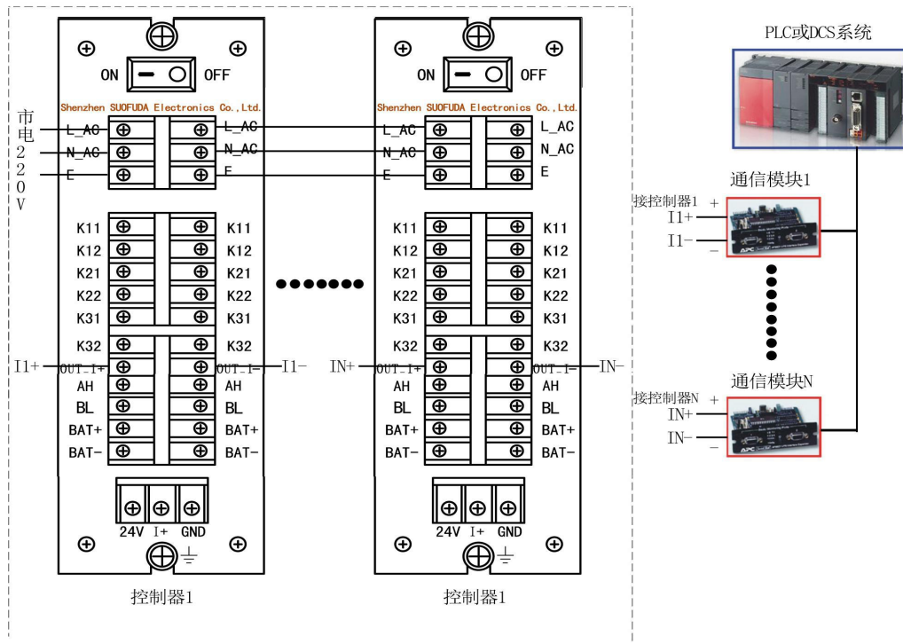
(图 15、报警控制器输出的 4-20mA 标准信号与 DCS 或 PLC 的连接方法)
