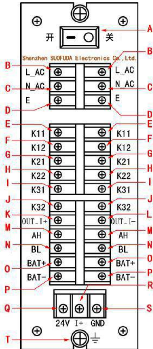
(图 3B、电源单元接线端子板)
